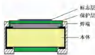
图 B.4 无引脚矩形片状元件示意图
