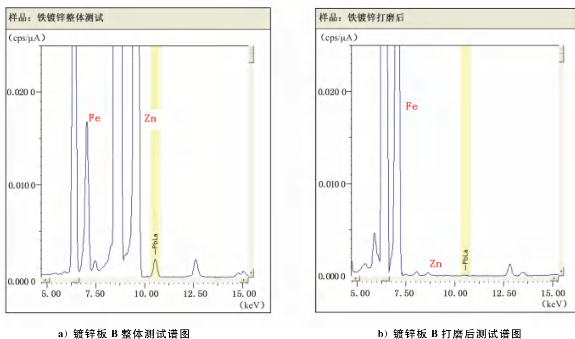
图 C.9 镀锌板 B 打磨前后测试谱图
